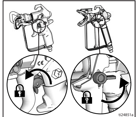
LineLazer ES 1000
