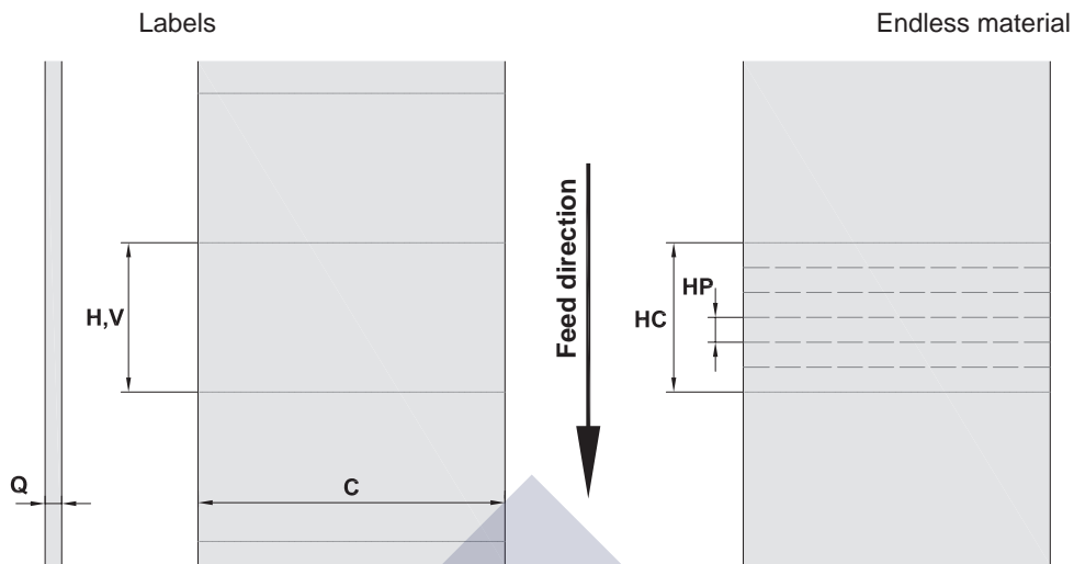
Fig. 17 Media dimensions
