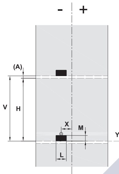
Fig. 19 Reflex mark dimensions
