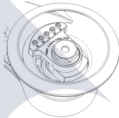
4. Machineconfiguratie voor gebruik in combinatie met beschermplaat of interface.
