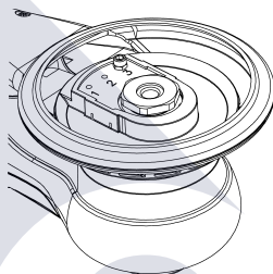
6. Конфигурација на машината за употреба со штитник за подлога или подметка.
