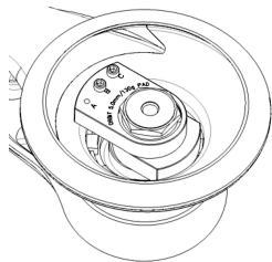
1. Konfiguracija uređaja prilikom raspakiranja.
