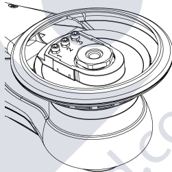
7. Конфигурација на машината за употреба со штитник за подлога или подметка.
