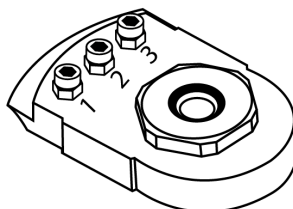
3. Maskinkonfigurasjon for bruk med beskyttelsesplate eller mellomskive, skruer og muttere montert i posisjon 1, 2 og 3.
