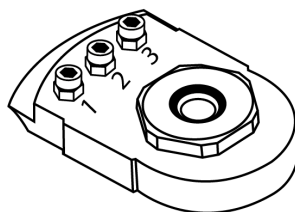
3. Konfiguration der Schleifmaschine für die Verwendung einer Schutz- oder Softauflage, Schrauben und Muttern in den Positionen 1, 2, 3 installiert.
