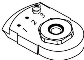
2. Конфигурация на машината за използване с предпазител за подложката или интерфейс, с винт и гайка, поставени на позиция 3.
