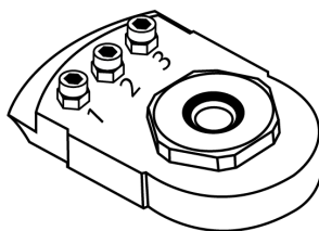
3. Maskinkonfiguration för användning med pad saver eller slipplatta, skruvar och muttrar monterade i hål nr 1, 2 och 3.
