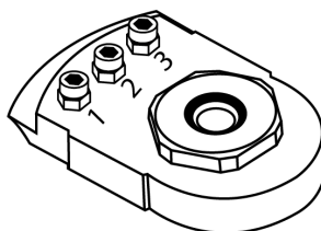
3. Kvörðun verkfærisins til notkunar með skífuhlíf eða millistykki, skrúfur og rær settar upp í 1., 2. og 3. stöðu.
